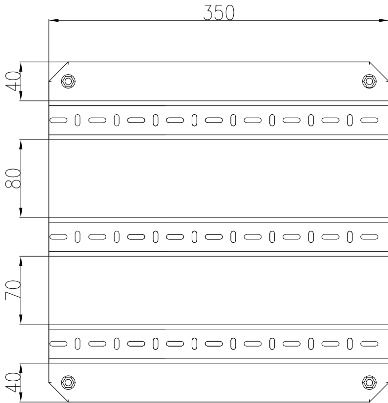
VISTA FRONTAL DETALLE DE RIELES
